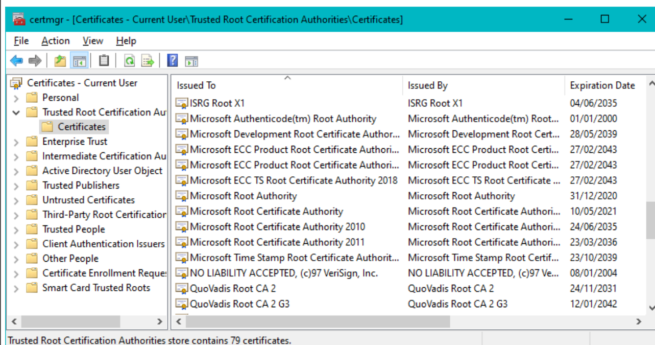
Abbildung 1. Windows 10 Zertifikat-Manager
