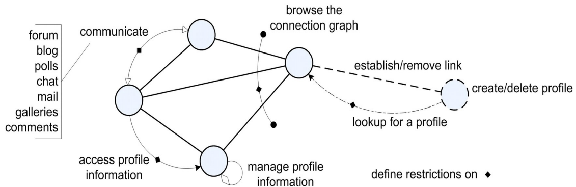
Figura 3: Principali funzionalità di una tipica piattaforma di social networking ( https://hal.archives-ouvertes.fr/hal-00687145 )
