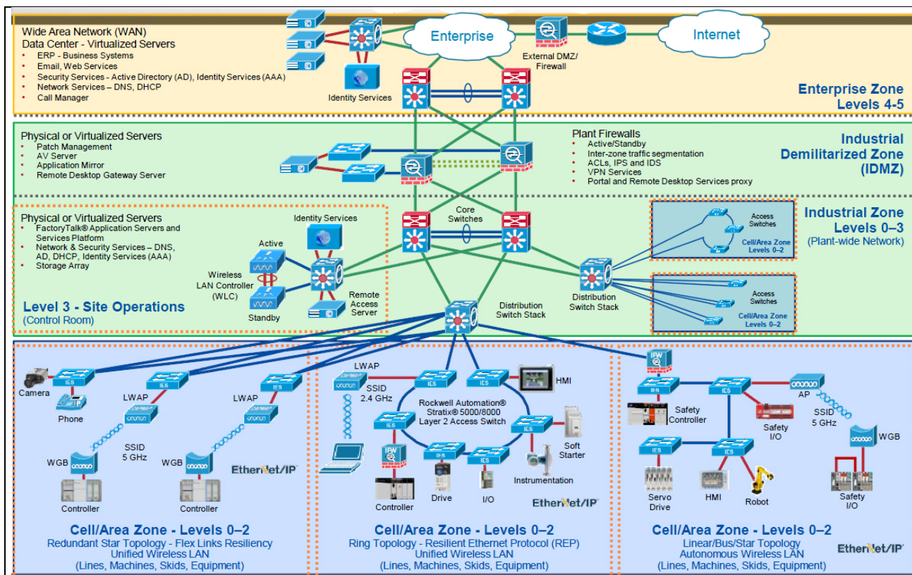
Fig. 5: IDMZ
